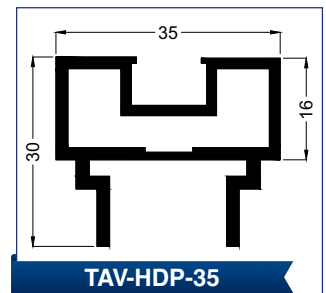
Horizontal Door Profile
