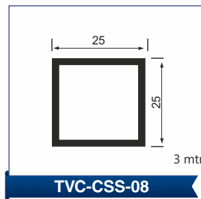
TVC-CSS- LEG
